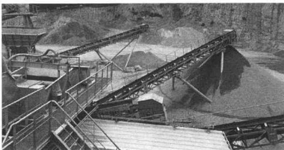
Ensemble de convoyeur pour l'exploitation de carrières. © Groupe Garonne
